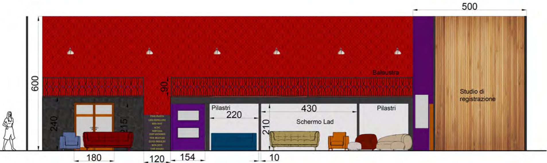
SEZIONE B-B
