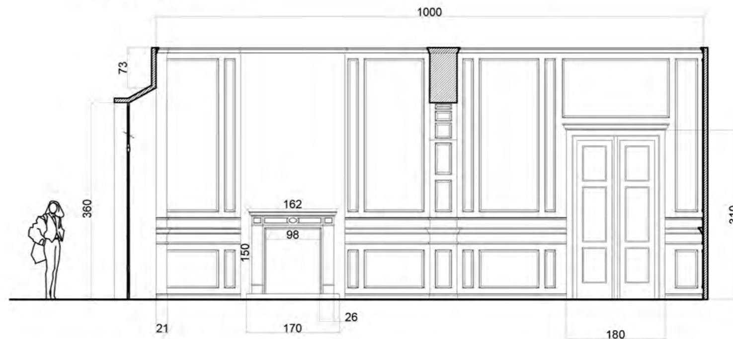
Prospetto B-B'
