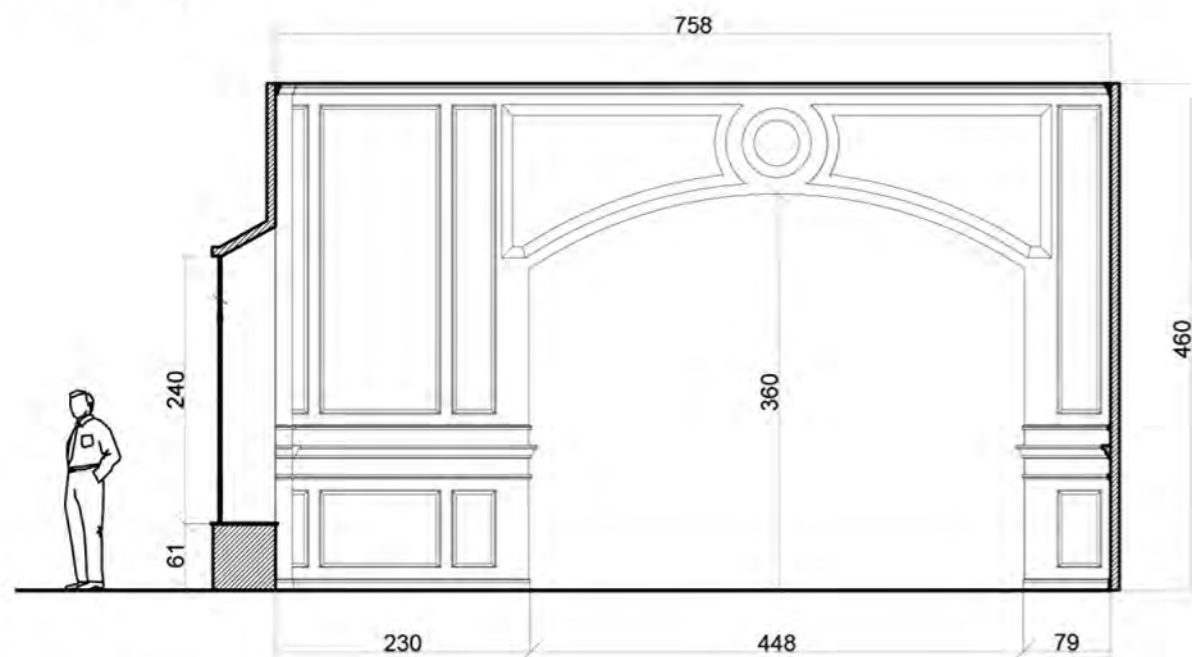
Prospetto D-D'
