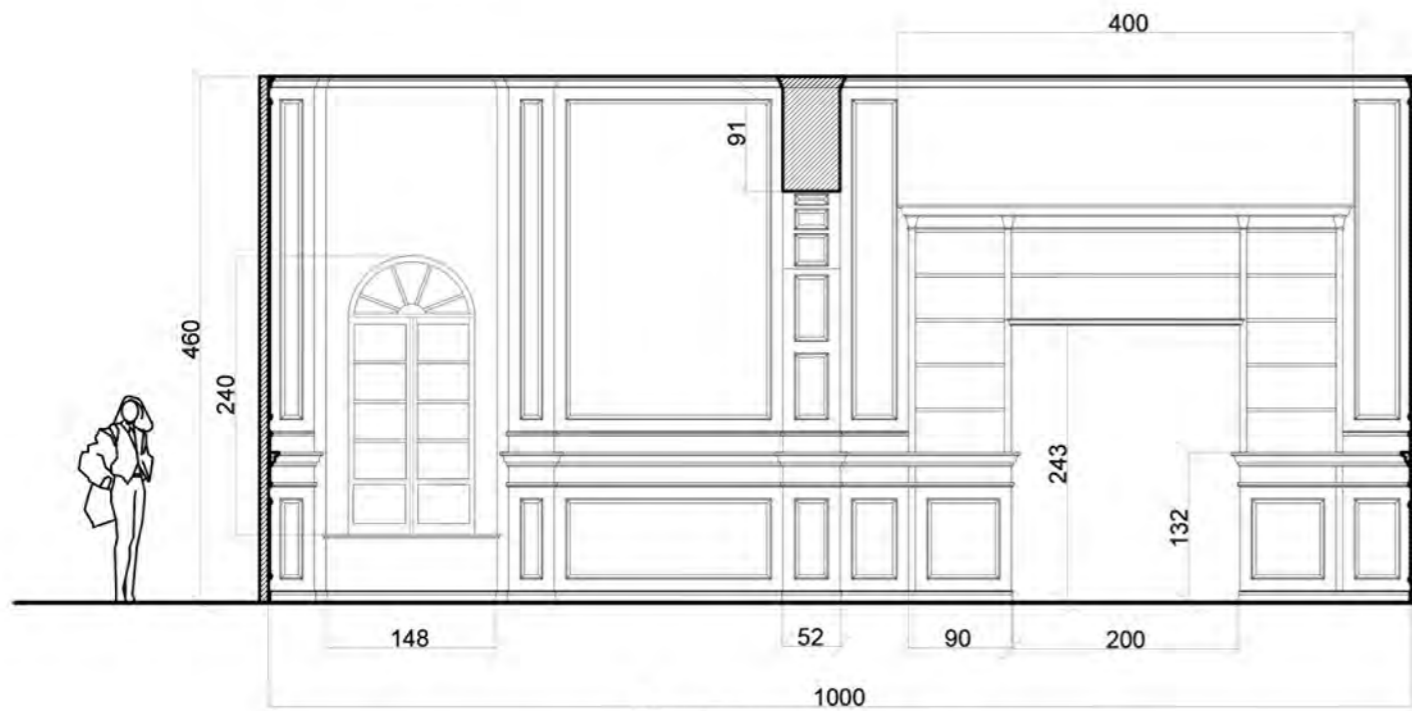
Prospetto C-C'
