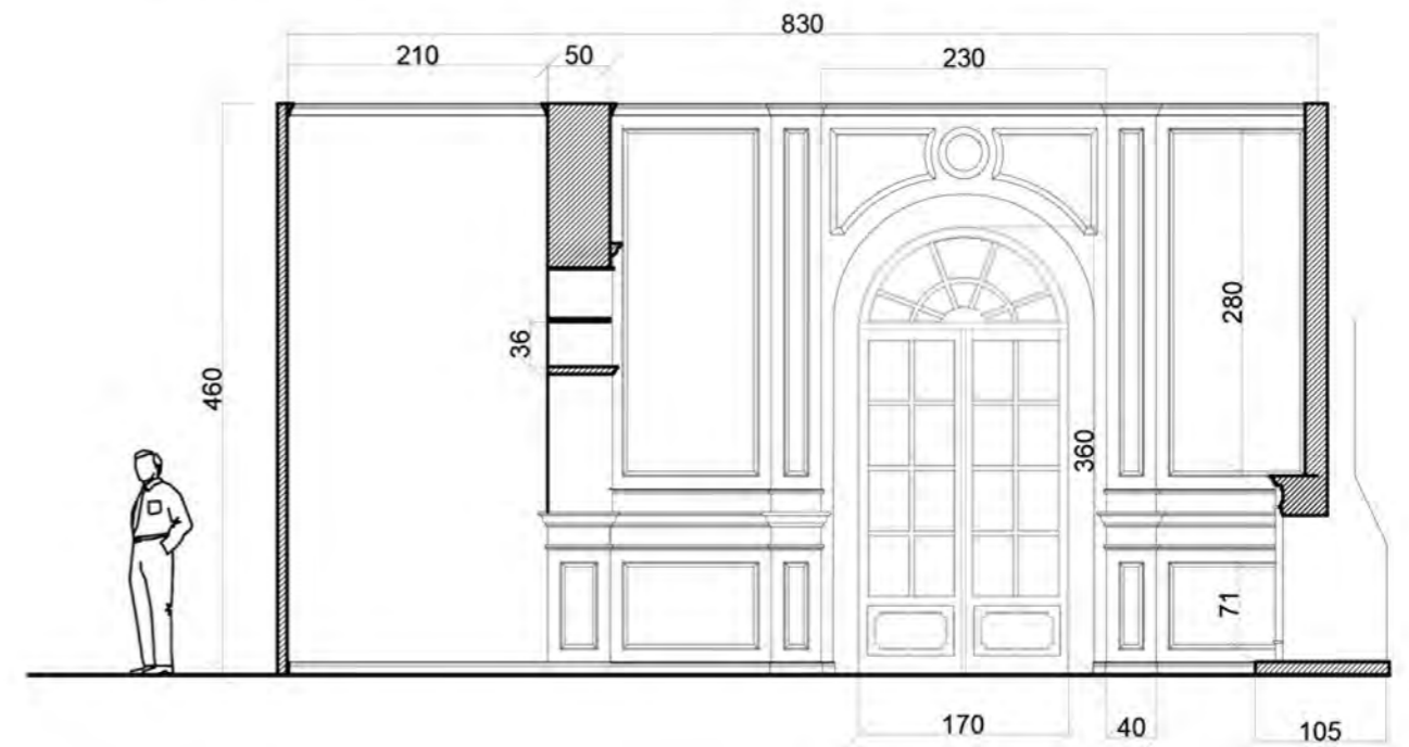
Prospetto A-A'
